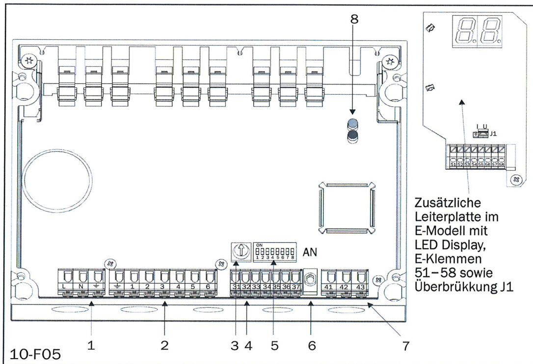
Fig. 5 Anordnung der Anschlussklemmen u.a.
